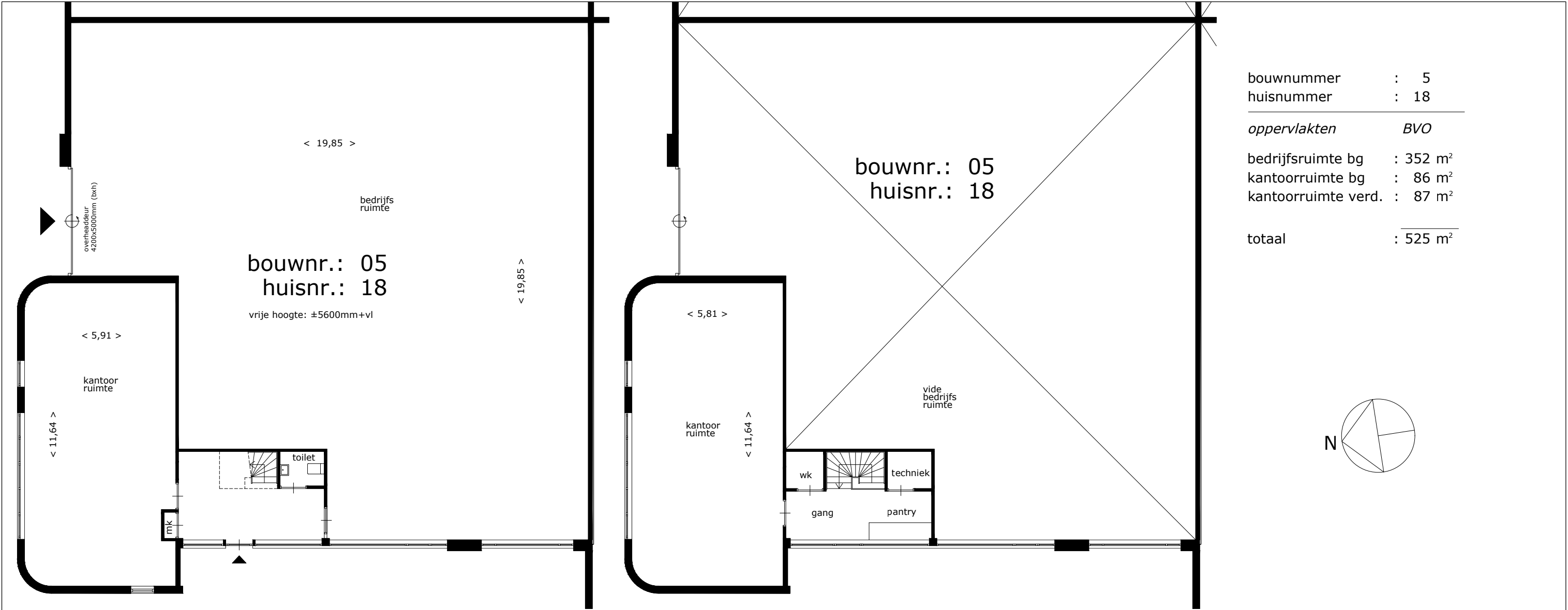
begane grond
